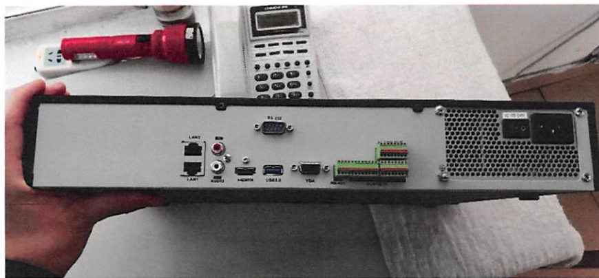
硬盘录像机背部接口
