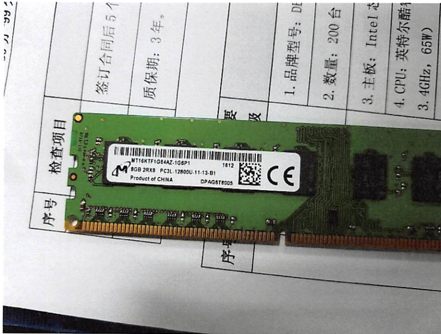
内存铭牌
