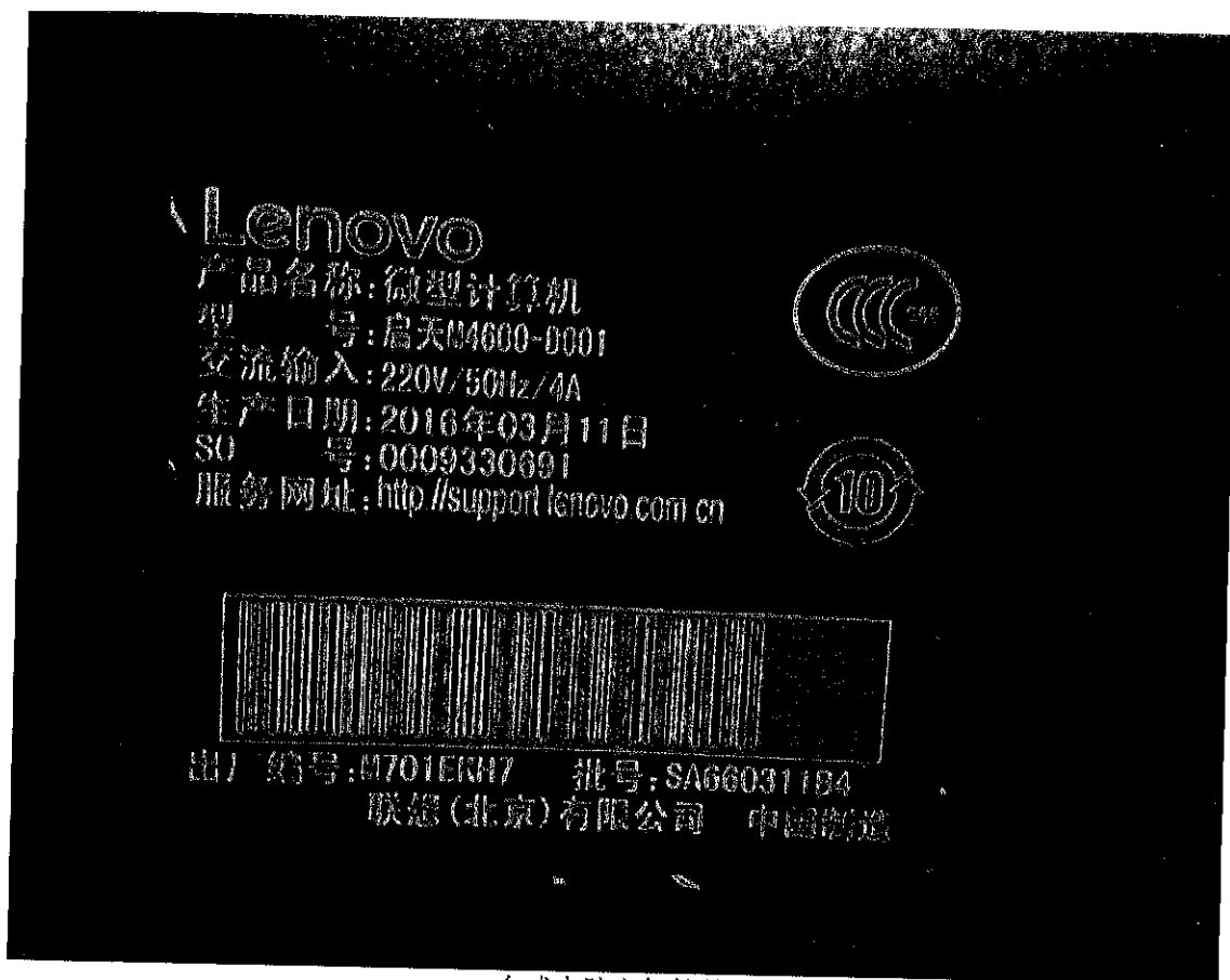
台式电脑主机铭牌
