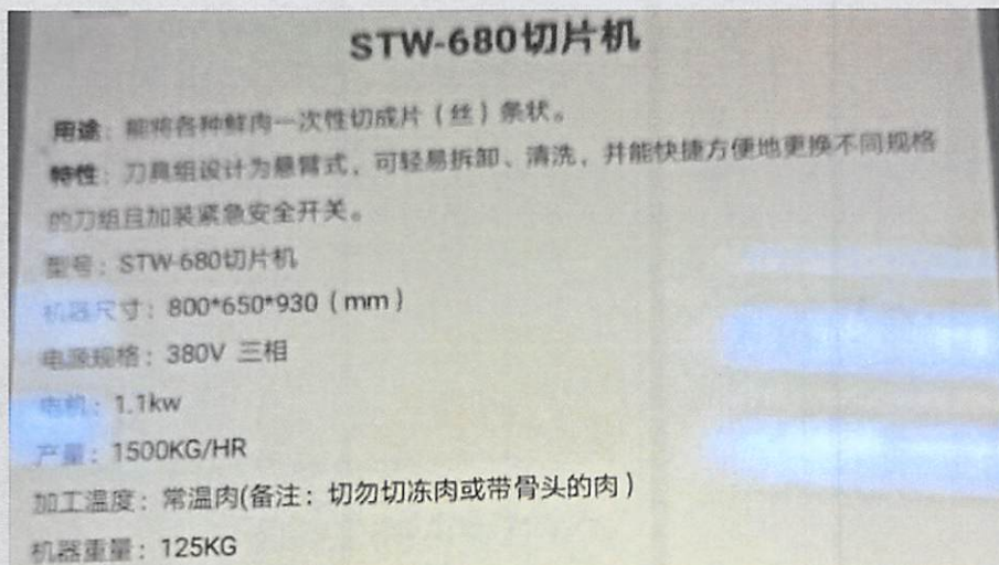
切片机主要技术参数
