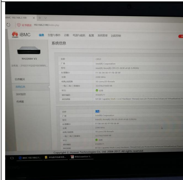
系统信息
