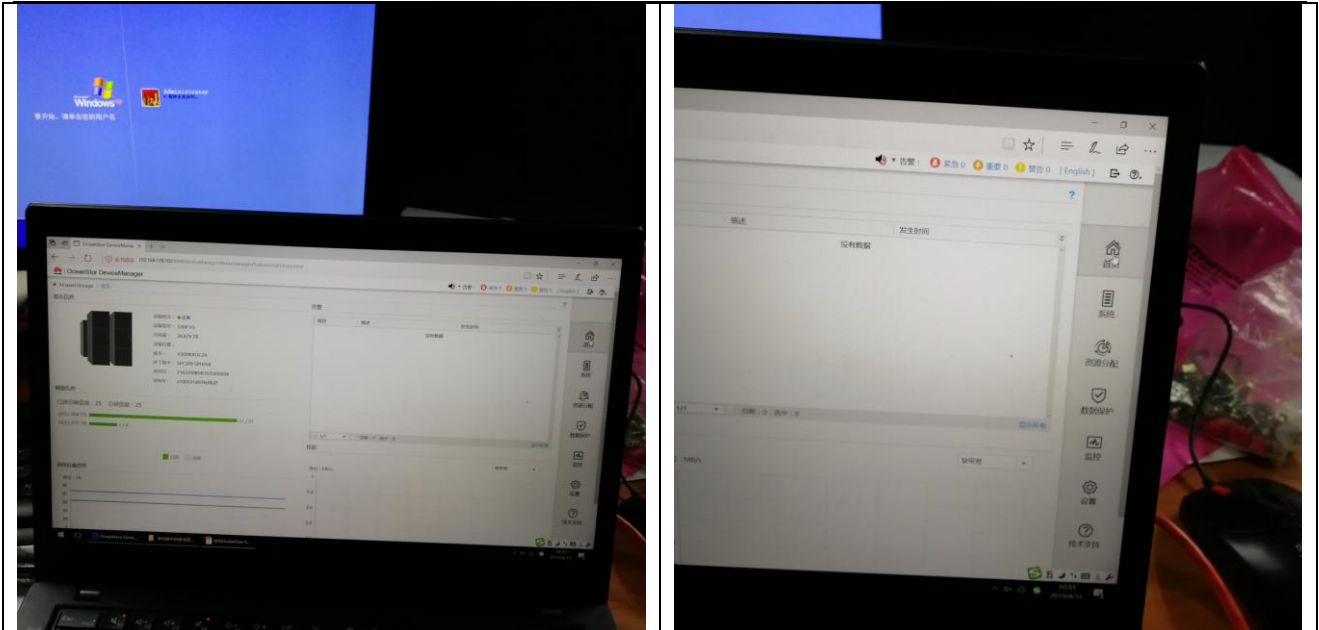
图形化管理
