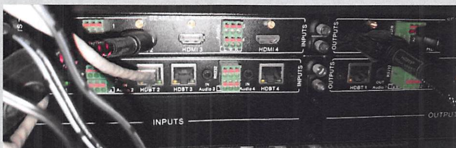
8 进 8 出混合拼接矩阵输入、输出卡
