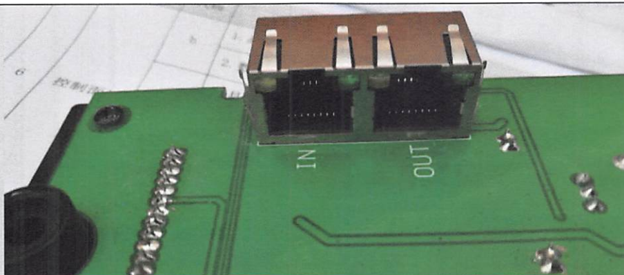
控制面板接口
