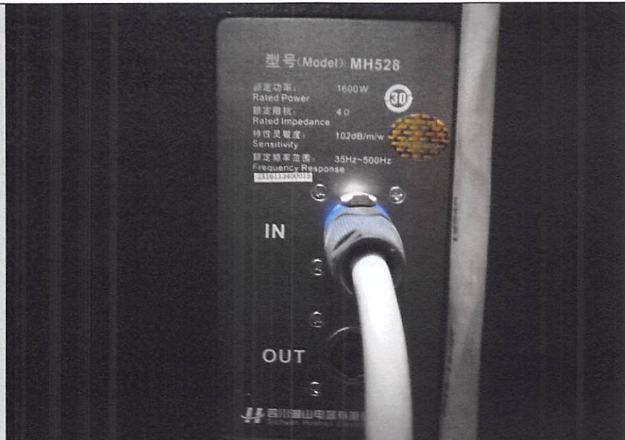
超低音扬声器铭牌
