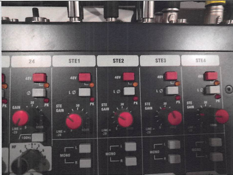
专业调音台 2 48V 幻象电源开关
